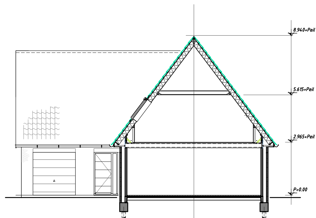
doorsnede hoofdbouw
