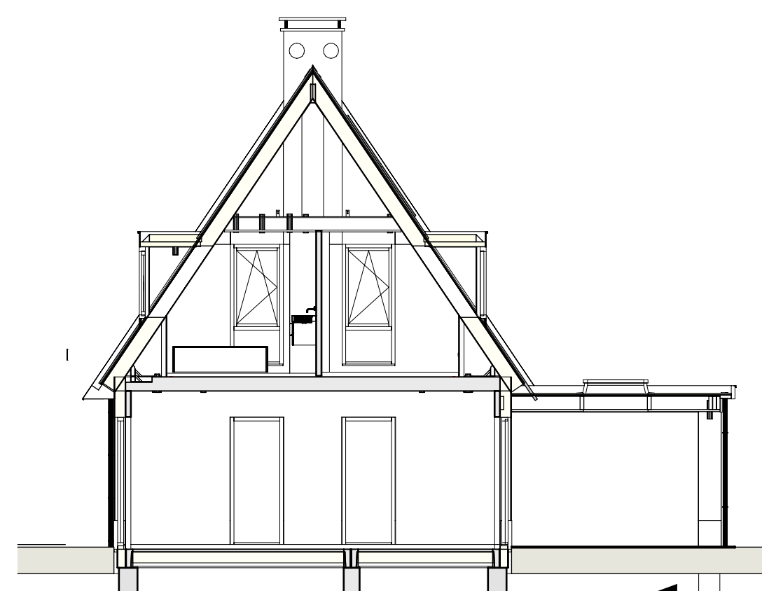
Dwarsdoorsnede
