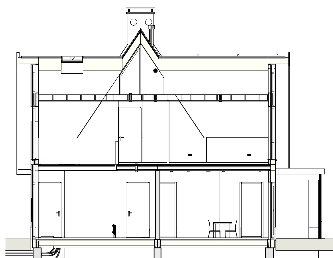
Dwarsdoorsnede
