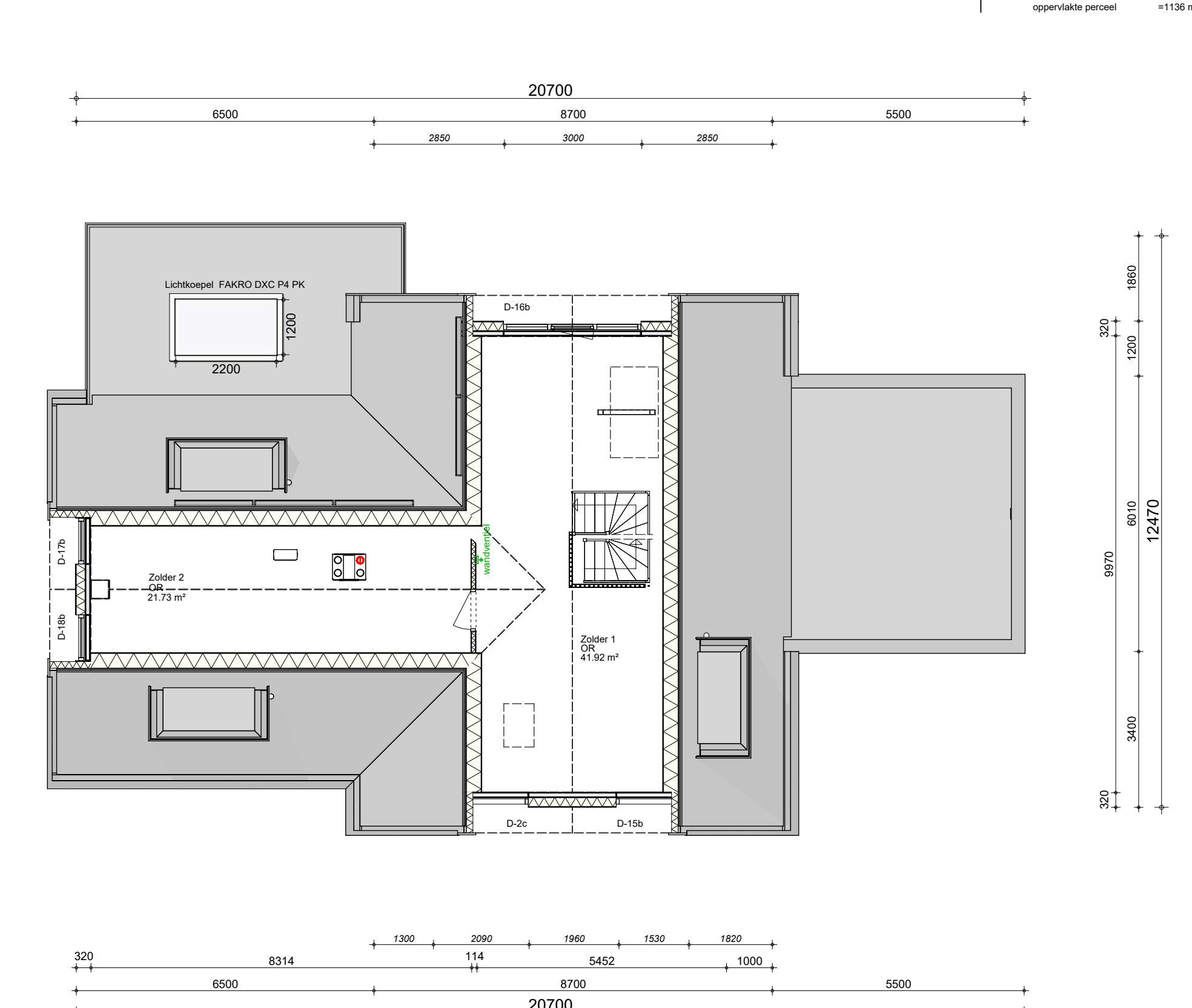
2e Verdieping
