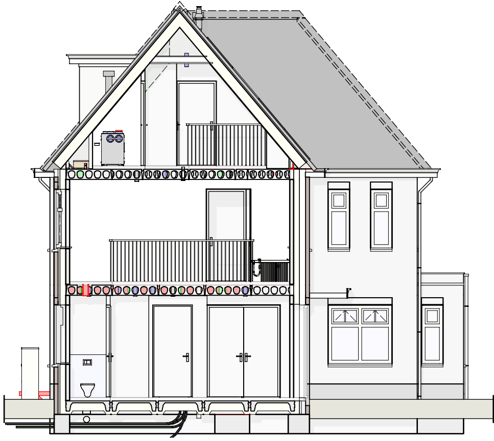
Dwarsdoorsnede
