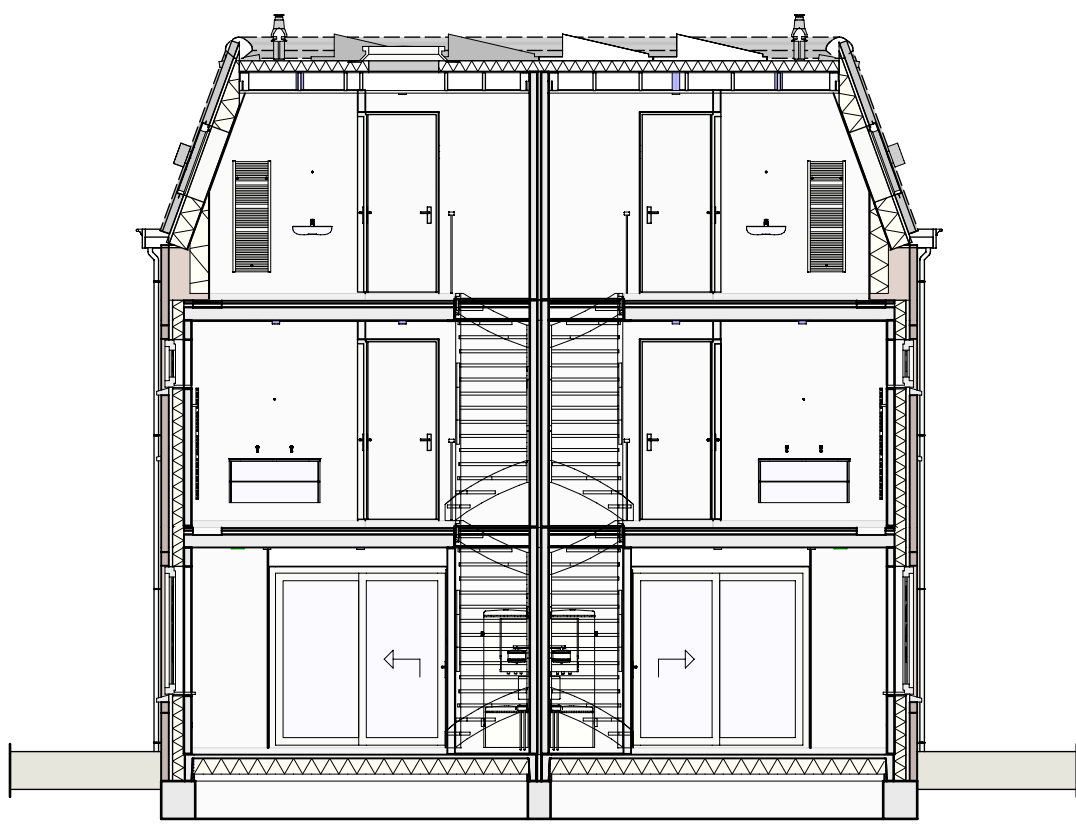
Doorsnede
