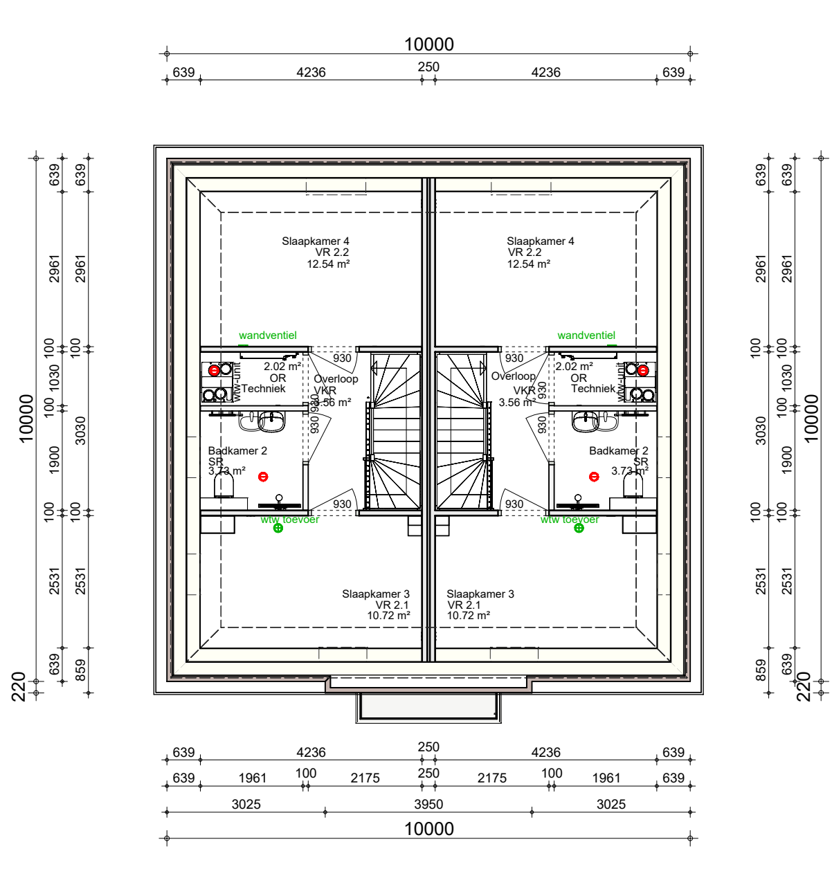
2e Verdieping
