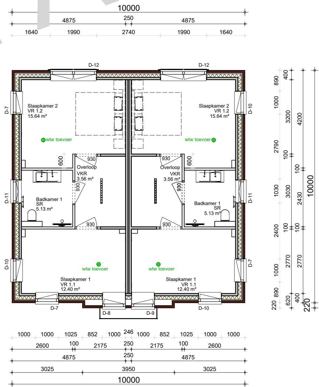
1e Verdieping
