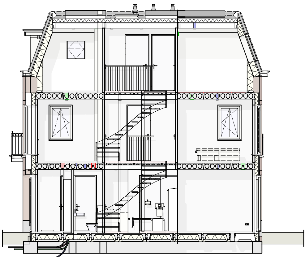
Doorsnede
