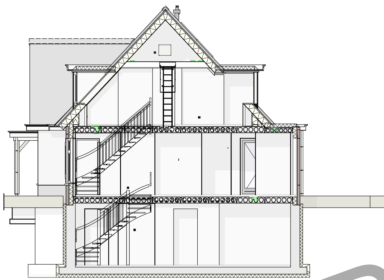
Doorsnede
